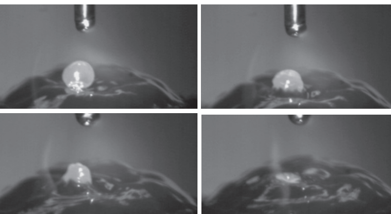
MAG welding
